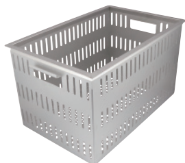
18-8 軽量ステンレスコンテナ 底面高通気タイプ ST-1A290 上代：30,000 CD：SA2240 外寸：515×340×H290mm 材質：SUS304 2B仕上げ 板厚：0.6mm
