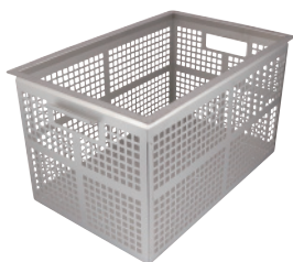
18-8 軽量ステンレスコンテナ 側面高通気タイプ ST-2A290 上代：31,000 CD：SA2241 外寸：515×340×H290mm 材質：SUS304 2B仕上げ 板厚：0.6mm
