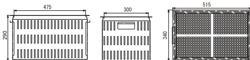
18-8 軽量ステンレスコンテナ 側面高通気タイプ ST-2A290 上代：31,000 CD：SA2241 外寸：515×340×H290mm 材質：SUS304 2B仕上げ 板厚：0.6mm
